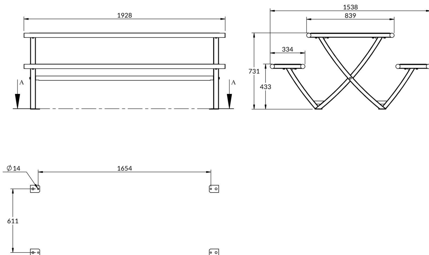
COUPE A-A
